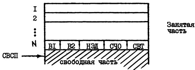
Рис.4. Начальные установки перед отождествлением уровней скобочных структур и структура стека переходов
